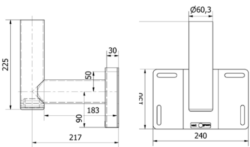
Vinkelfäste 60
